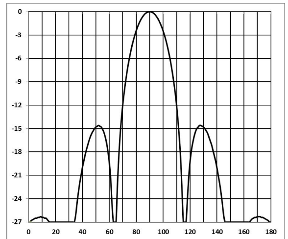
Диаграмма направленности в вертикальной плоскости
