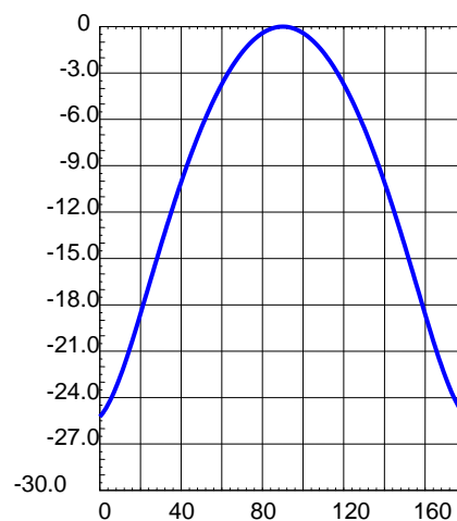
Диаграмма направленности в вертикальной плоскости
