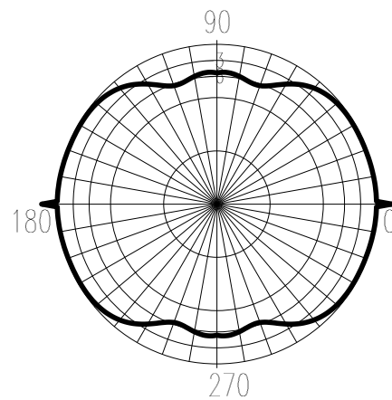
Диаграмма направленности в горизонтальной плоскости
