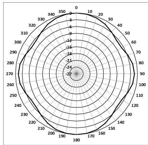
Диаграмма направленности в горизонтальной плоскости
