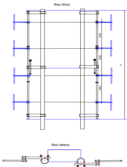
Внешний вид антенны
