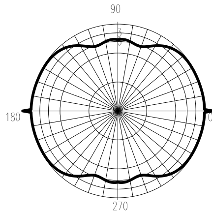
Диаграмма направленности в горизонтальной плоскости
