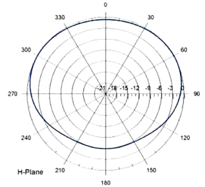
Диаграмма направленности в горизонтальной плоскости
