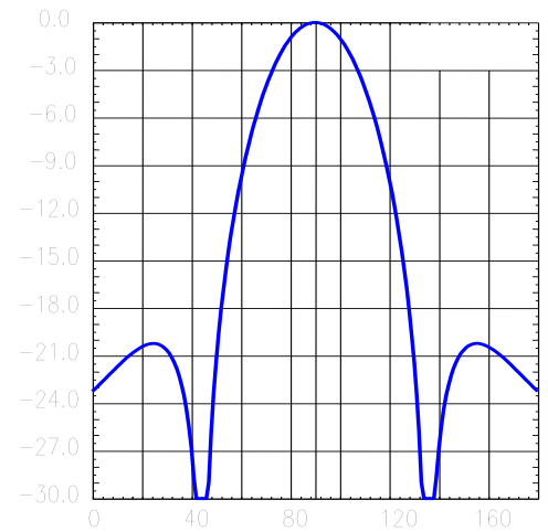
Диаграмма направленности в вертикальной плоскости
