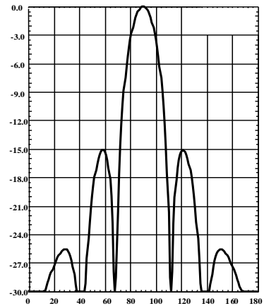
Диаграмма направленности в вертикальной плоскости
